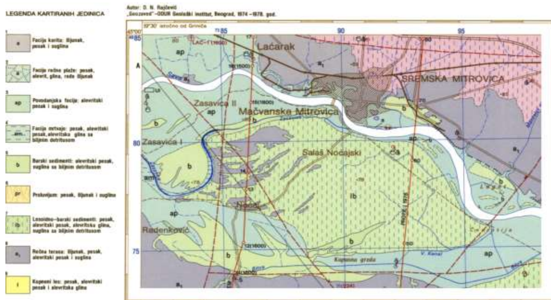
Илустрација 2 - Основна геолошка карта СФРЈ. Лист Шабац, Л-34-112 (1983)
