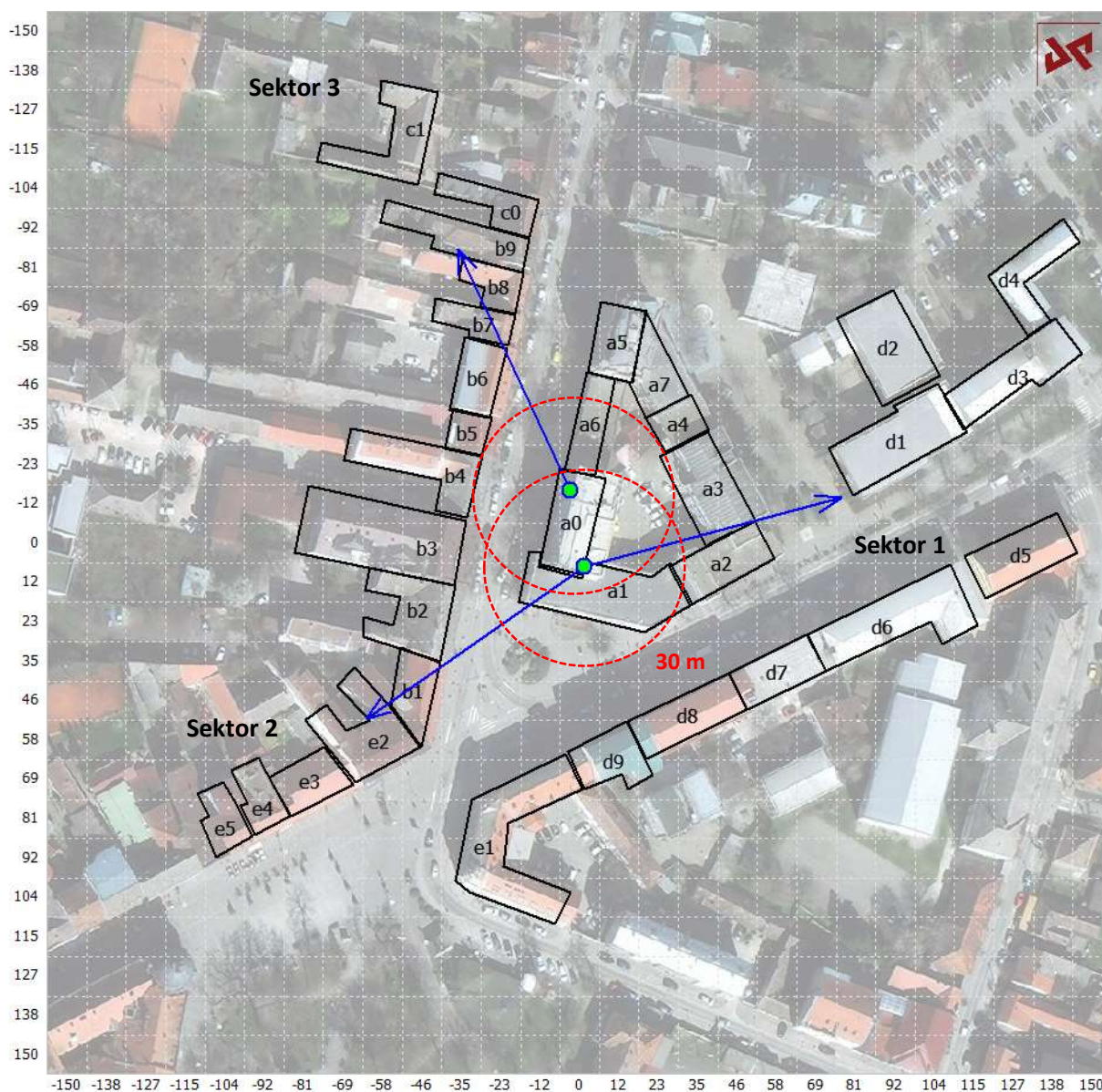
Slika 2.5 Prikaz pravaca zračenja antena bazne stanice i pozicije okolnih objekata
