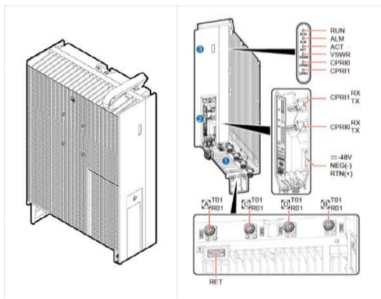
Slika 3.6 RRU5502 jedinica
